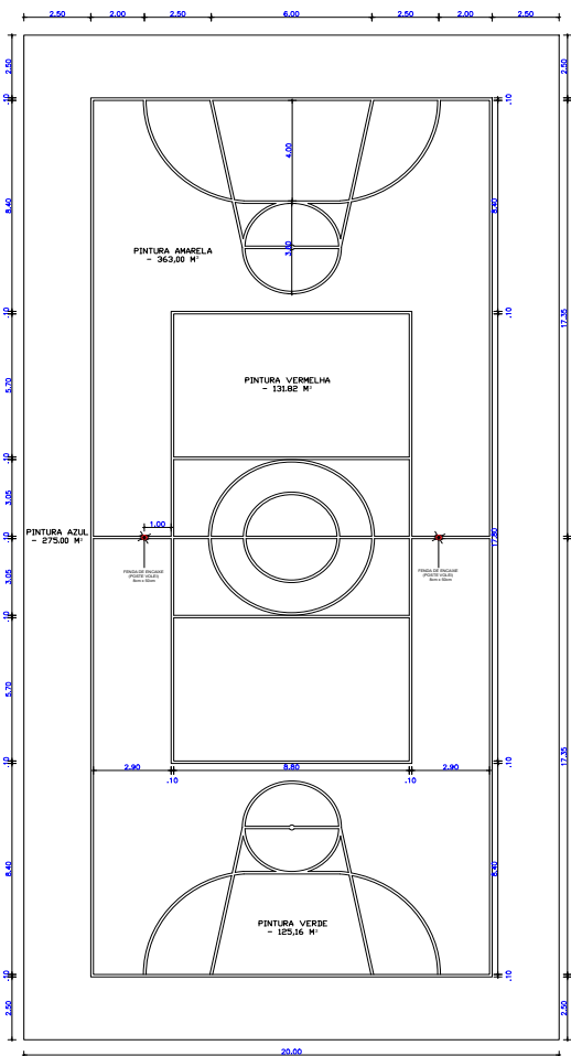
DIAGRAMA DE PINTURA 1:100
