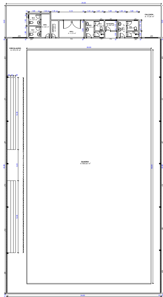
PLANTA BAIXA 1:100
